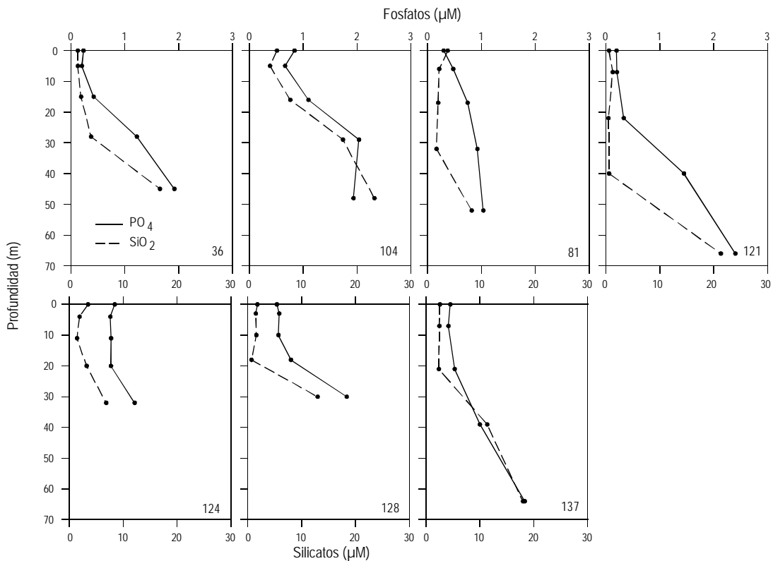
Figura 3. Distribuciones verticales de PO_4 (—) y SiO_2 (---) en las estaciones de muestreo. Figure 3. Vertical distribution of PO_4 (—) and SiO_2 (---) at the sampling stations.
