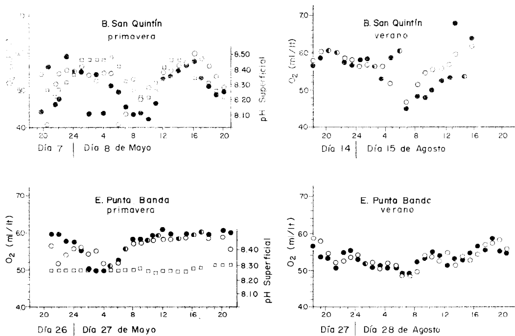
Fig. 4.- Variación de oxígeno disuelto y pH en las bocas de San Quintín y el Estero. Círculos y cuadros claros representan valores de superficie y los oscuros de fondo. Los cuadros representan valores
