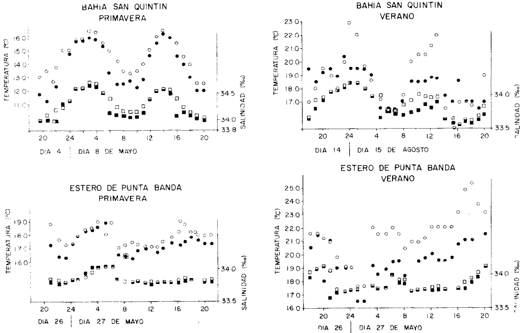
Fig. 2.- Variación de temperatura y salinidad en las bocas de San Quintín y el Estero. Círculos claros representan valores de superficie y los oscuros de fondo. Los círculos representan temperatura.
