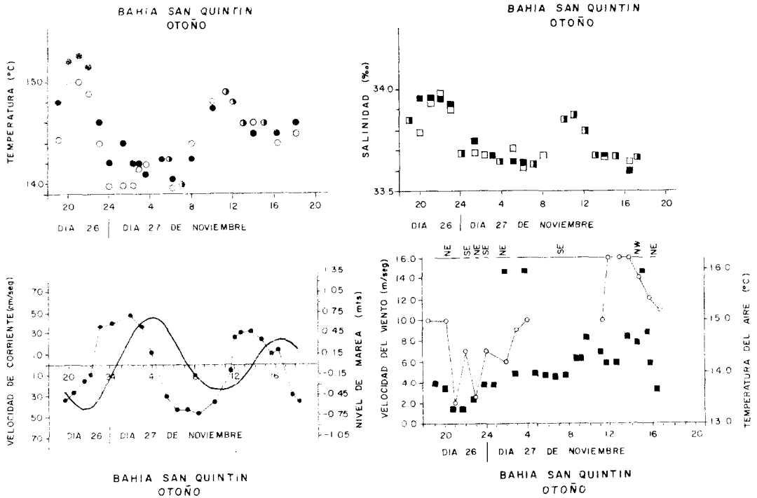
Fig. 3.- Variación de temperatura, salinidad, velocidad de corrientes, marea, velocidad del viento y temperatura del aire en la boca de San Quintín en el muestreo de otoño. Círculos claros representan valores de superficie y los oscuros de fondo, en las gráficas de T°C y S‰/oo. La línea continua es la gráfica de marea. Círculos claros representan la velocidad del viento.
