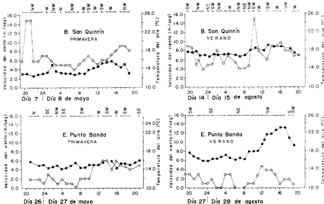
Fig. 5.- Variación de la velocidad del viento y la temperatura del aire en San Quintín y el Estero. Círculos claros representan la velocidad del viento y los oscuros la temperatura.
